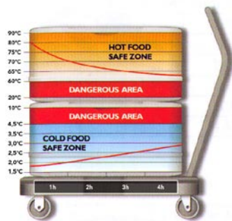
Temperaturkurven heiß & kalt im Zeitablauf.
